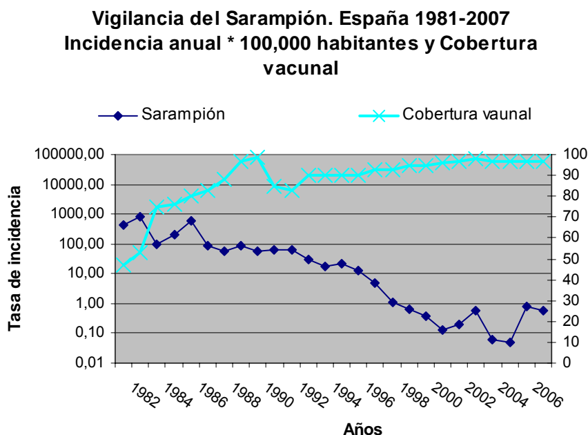
Gráfica 1: Incidencia de sarampión y coberturas vacunales medias en España desde 1981 hasta 2007.
