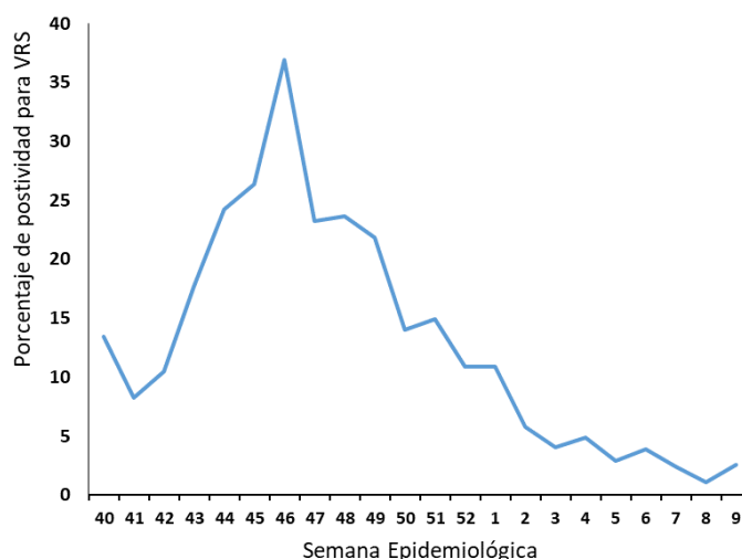
Figura 10. Porcentaje de positividad de VRS. Sistema no centinela. Temporada 2021-22. España
