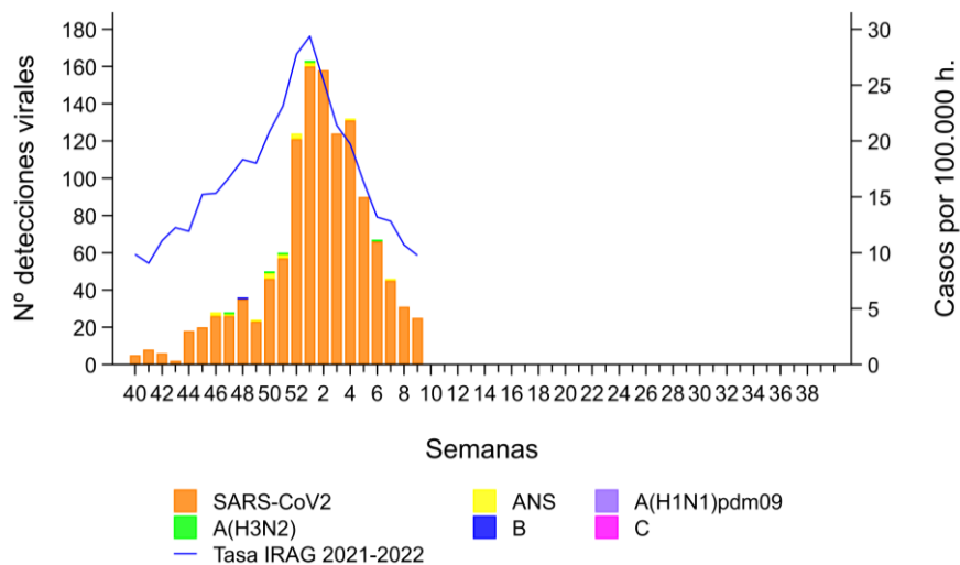
Figura 4. Tasas de incidencia semanal de IRAG y nº de detecciones SARS-CoV-2 y gripe. Vigilancia centinela de IRAG. SiVIRA, temporada 2021-22. España
