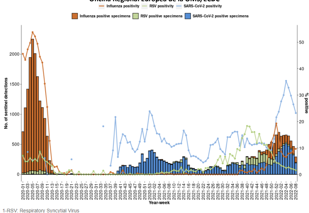
Figura 13. COVID-19, gripe y VRS. Detecciones procedentes de muestras centinela en AP. Oficina Regional Europea de la OMS/ECDC
